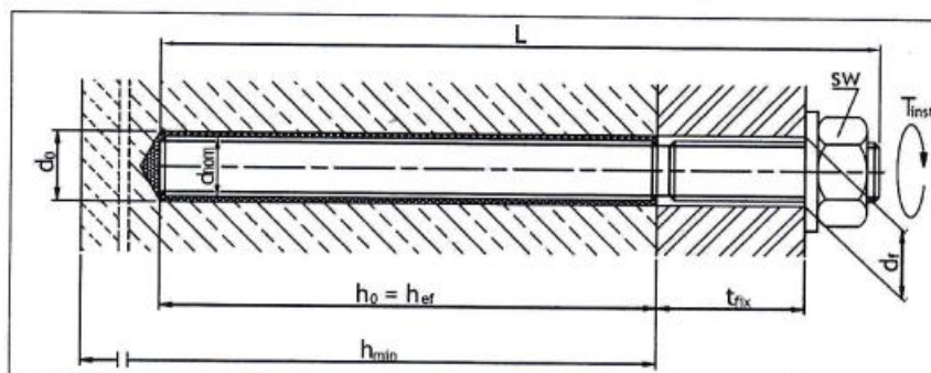
Рис. 6. Размеры и функциональные параметры стальных стержней
