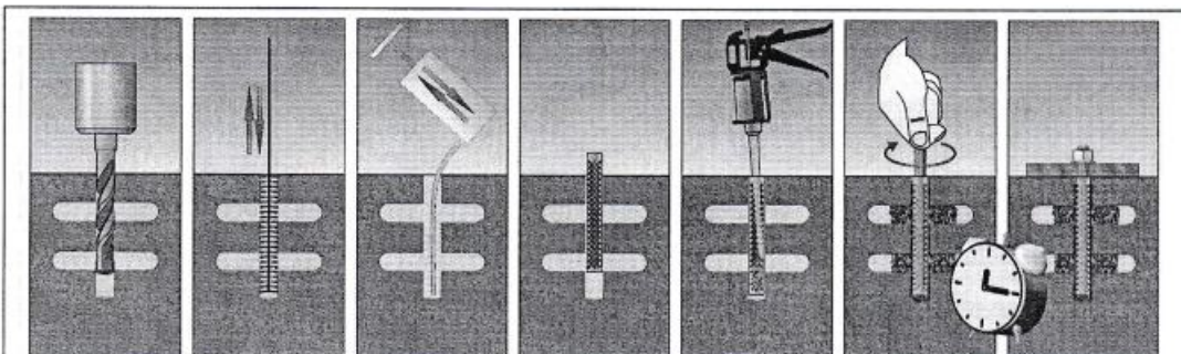
Рис. 8. Установка клеевых анкеров в пустотелые материалы
