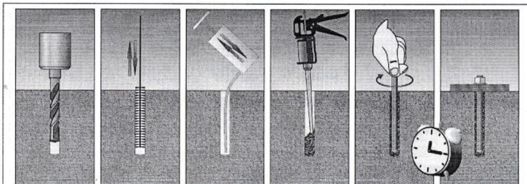
Рис. 7. Установка клеевых анкеров в полнотелые материалы
